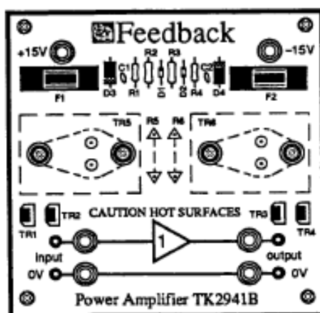
Εικ. 1.2 Ο Ενισχυτής Ισχύος TK2941B
