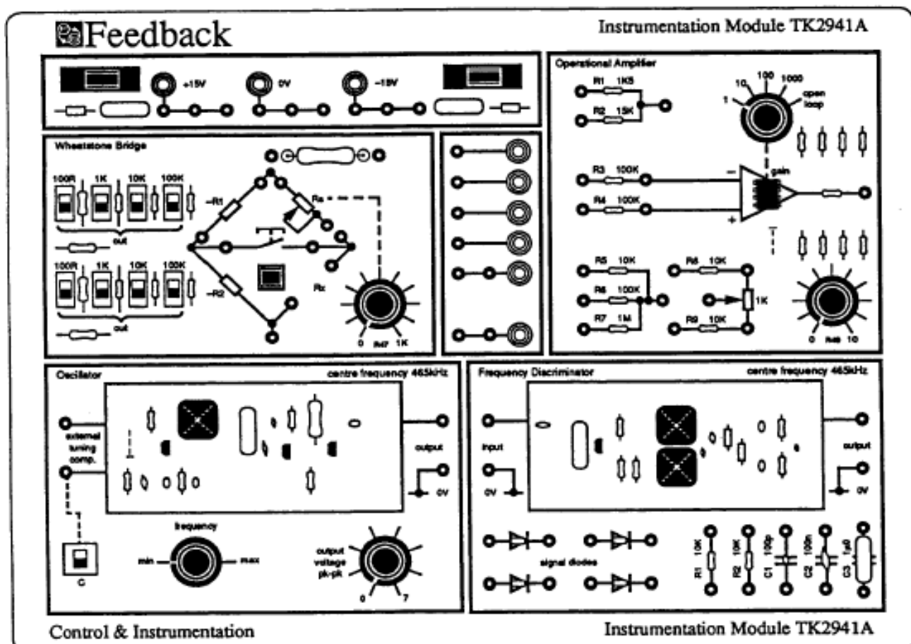
Εικ. 1.1 Η Μονάδα Οργάνων TK2941A
