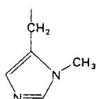
Anserine
